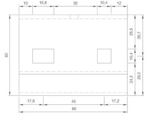
Ansicht Doppelagraffe justierbar/fixierbar
