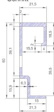
Schnitt
