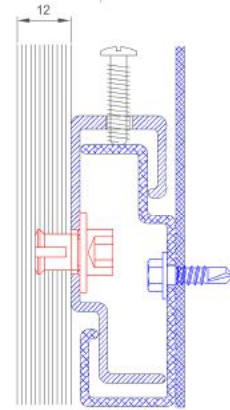
Keil Dübelhülse TERGO Keil U-Scheibe 6,4 Keil Zylinderkopfschraube M6x12
