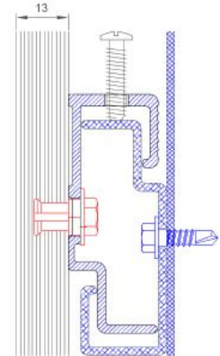
Keil KH AA 8,5 Keil Sechskantschraube M6x13 555 020 809
