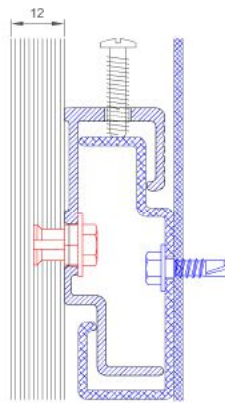
Keil KH AA 7 Keil Sechskantschraube M6x10 555 020 804
