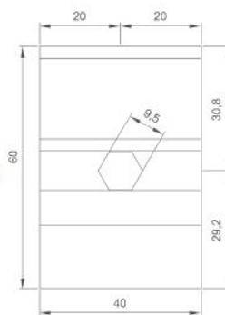
Ansicht
