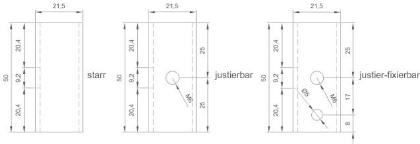
Draufsicht
