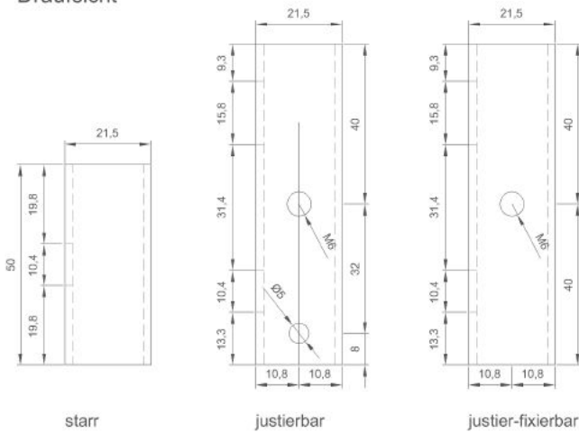
Draufsicht
